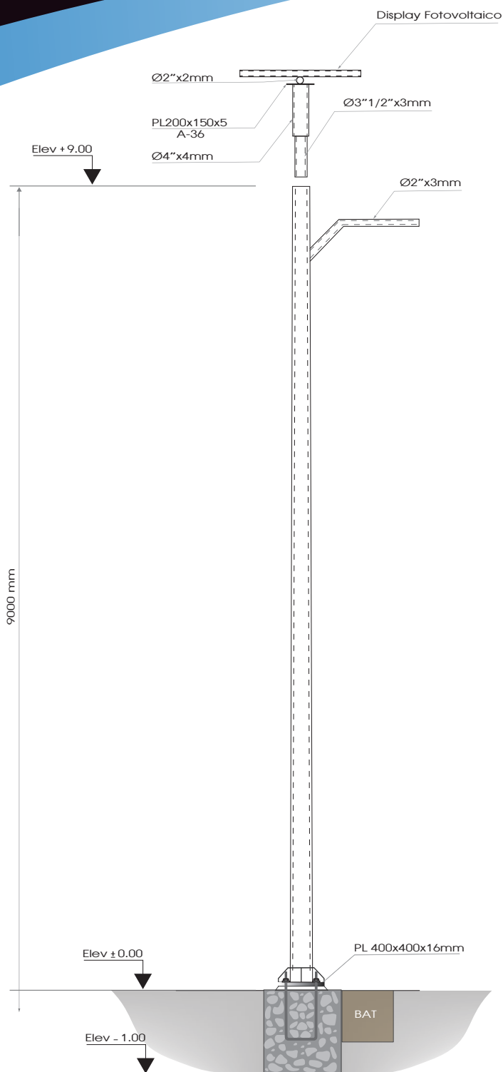
Elevación Poste Solar
